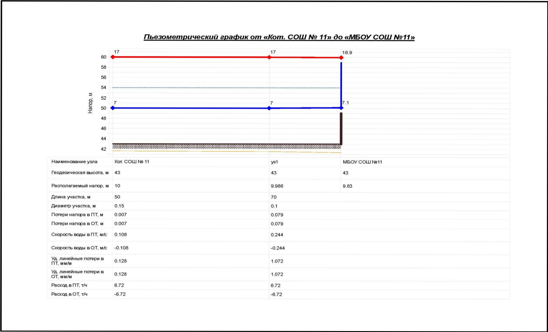
Рисунок 1.3.8.2 – Пьезометрический график Котельной СОШ № 11, ст. Григорьевская
