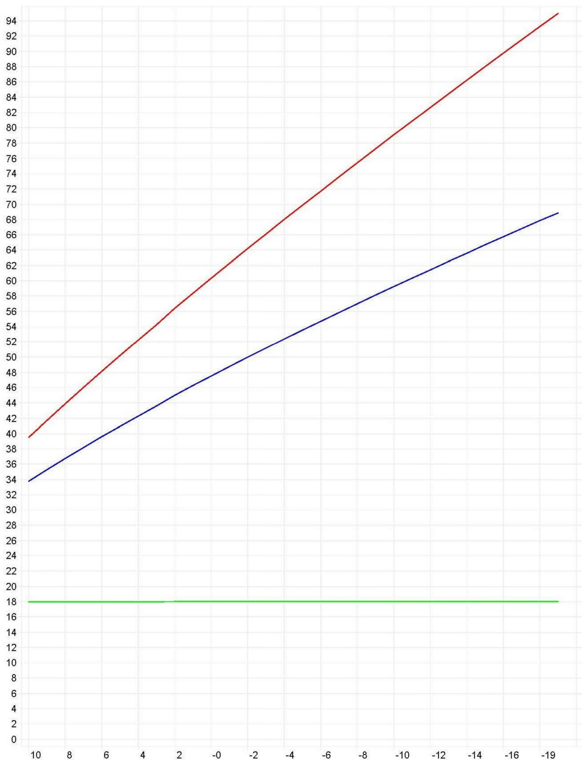
Температурный график котельных Григорьевского с.п.
